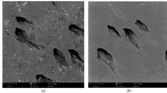
شکل ۶- تصاویر SEM بدست آمده قبل و بعد از فرآیند پلیمریزاسیون پلاسما (440 ×) (a) چرم عمل آوری نشده، (b) چرم عمل آوری شده با پوشش پلاسما
