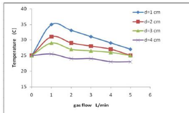
شکل ۹- بستگی دمای گاز به آهنگ شارش های کاز در فواصل مختلف
