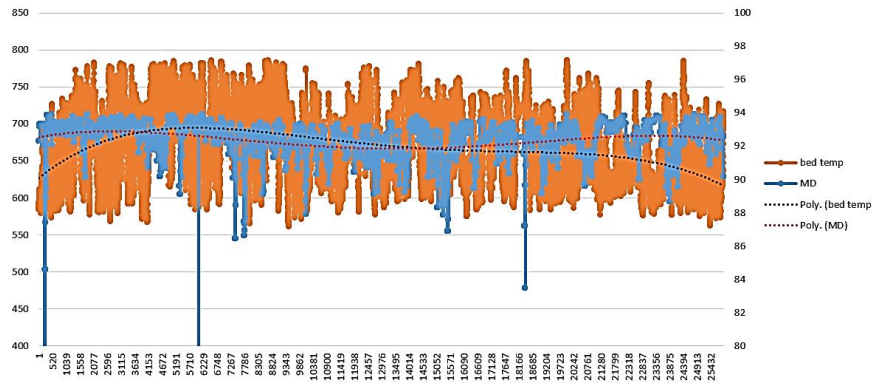
شکل ۶- کیفیت محصول و دمای بستر کوره احیا واحد گوهر شرکت توسعه آهن و فولاد گل گهر
