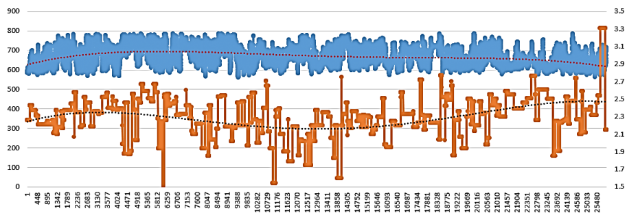
شکل ۷- دمای بستر کوره و میزان کربن خوروجی در واحد گوهر شرکت توسعه آهن و فولاد گل گهر
